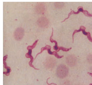
Fig. 1.14. Trypanosoma gambiense
